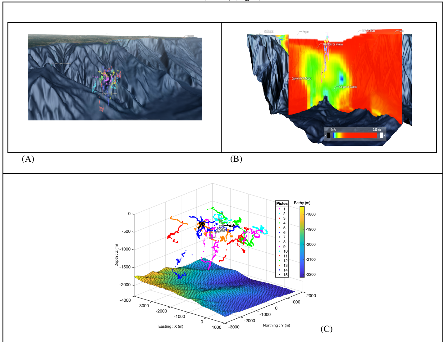
Figure 3 : Sondes 3D calculées par acoustique passive depuis la surface d'une meute de 6 cachalots au large du haut-fond Mejean, vers Monaco, le 2020.01.14 (A). (B) Ces prédateurs restent centrés 3h au centre d'un vortex, front océanique où est brassée une grande biomasse (Glotin et al. 2020). Ces vitesses de courants ont été calculées par Yann Oumières, MIO UTLN. (A,B) : Carte dynamique: http://sabiody.org/pub/SPHYRNA/3D/current_norm/ (C) : Vidéo: http://sabiody.org/pub/SPHYRNA/3D/SO_Glotin_Thellier_etal_PhyseterAlliance_Monaco_20200114_3DtracksX_Y_Z.mp4 (crédit H. Glotin)
